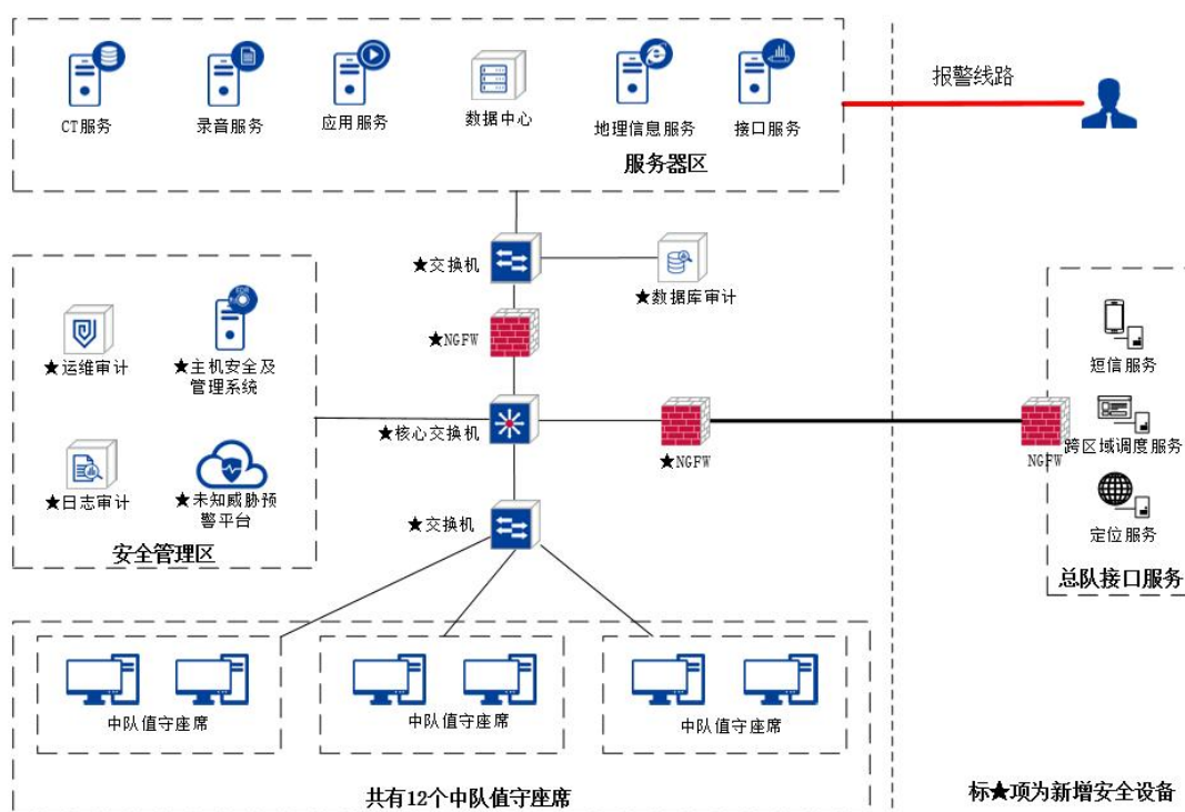
图 3 网络安全拓扑图
